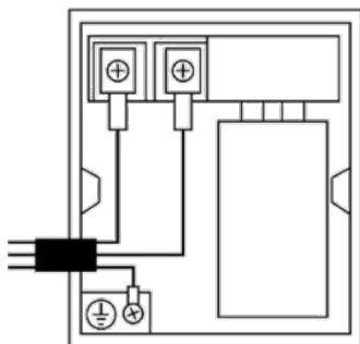
METODE DE CONECTARE LA REȚEAUA ELECTRICA
